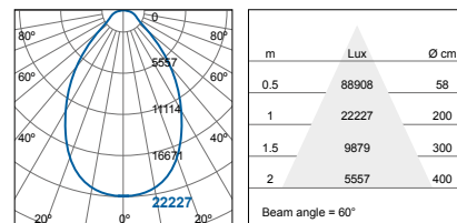
FFL74900v0-sc+060D-200W
