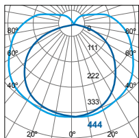
FIB75800v0 (4000K / 6500K)
