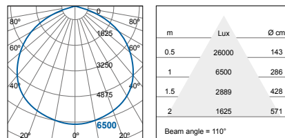
FHB71000v1-dc/ds+110D (115W) FHB71000v1-da+110D (115W)
