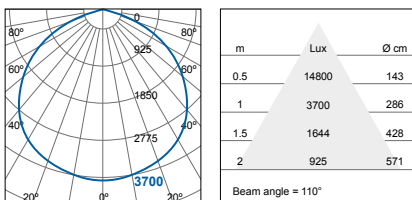
FHB71000v0-dc/ds+110D (70W) FHB71000v0-da+110D (70W)
