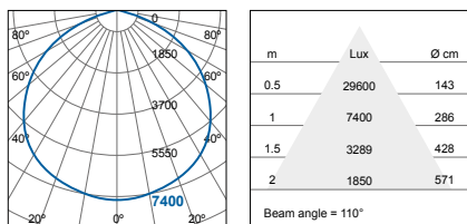
FHB71000v0-dc/ds+110D (150W) FHB71000v0-da+110D (150W)
