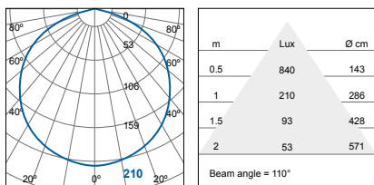
FIB76000v0-ps (4000K)
