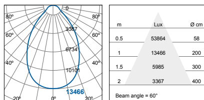
FFL74300v0-dssc+060D-120W FFL74300v0-ds+060D-120W
