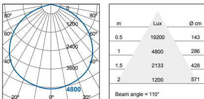
FHB71000v1-dc/ds+110D (80W) FHB71000v1-da+110D (80W)
