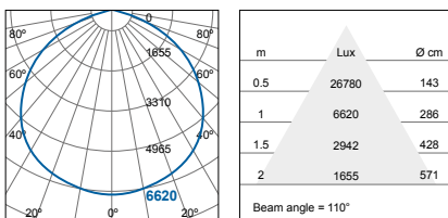
FHB71000v0-dc/ds+110D (125W) FHB71000v0-da+110D (125W)
