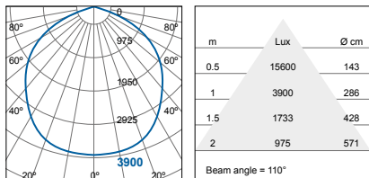
FFL71100v0
