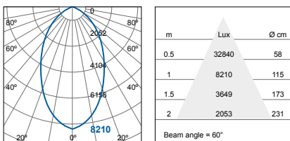
FHB71000v0-dc/ds+060D (70W) FHB71000v0-da+060D (70W)
